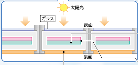
断面図
